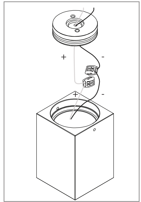
Cablare l'articolo Wire the article
